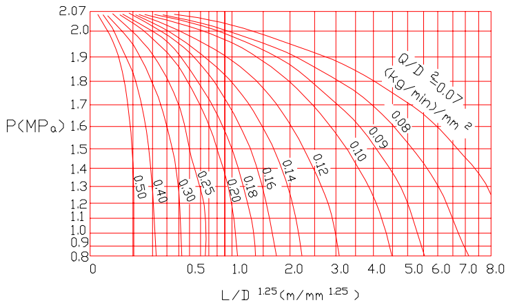
附图 C—2 低压系统管道压力降
