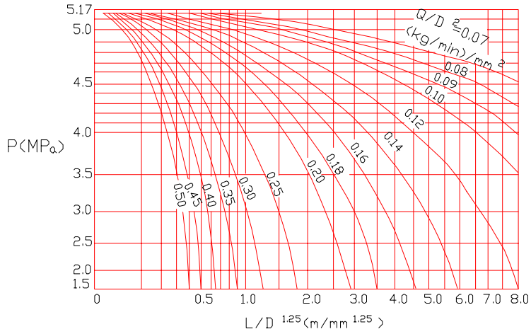
附图 C—1 高压系统管道压力降
